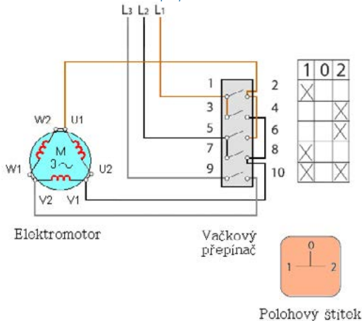
Obrázek 1.3 Schéma zapojení
