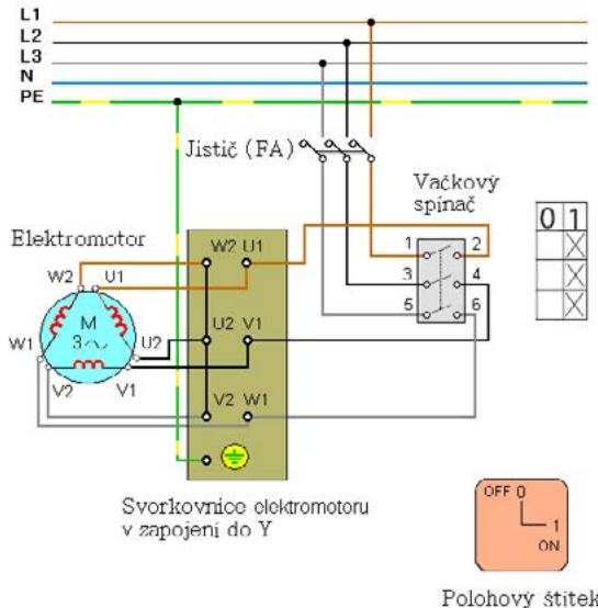
Obrázek 1.1 Schéma zapojení
