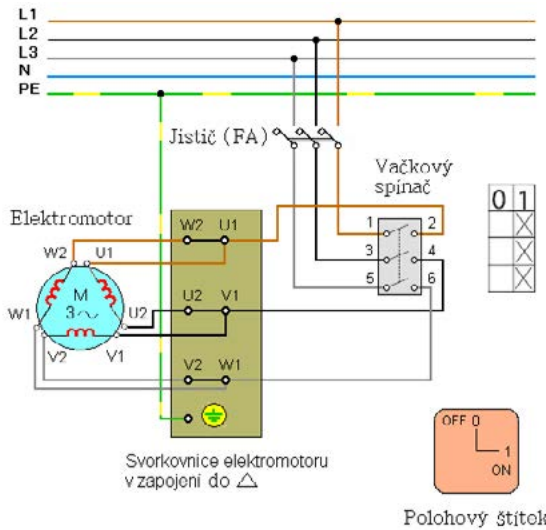
Obrázek 1.2 Schéma zapojení
